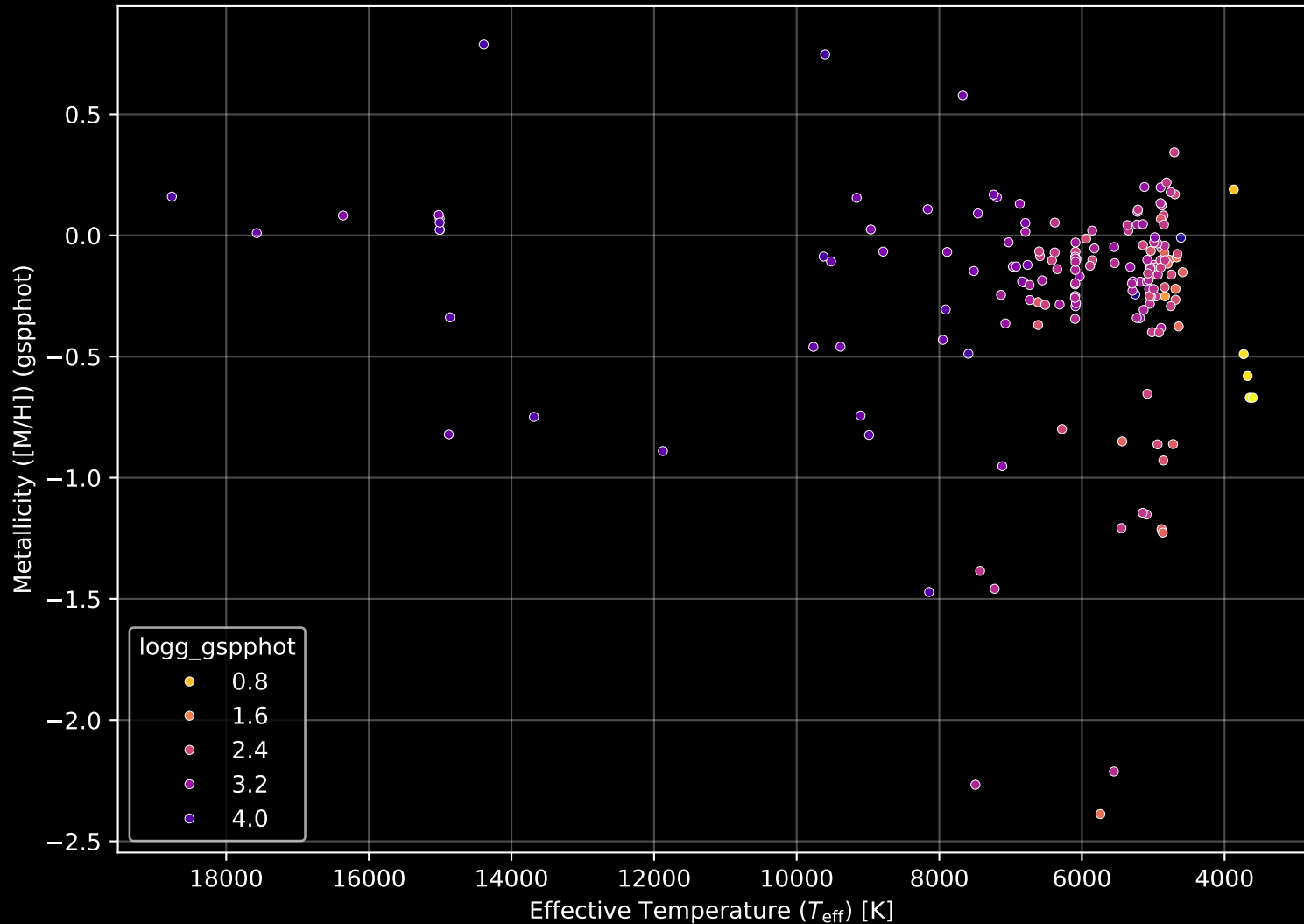
APOGEE DR17 Field: [109+04] Stellar Population Parameters (n= 172)
